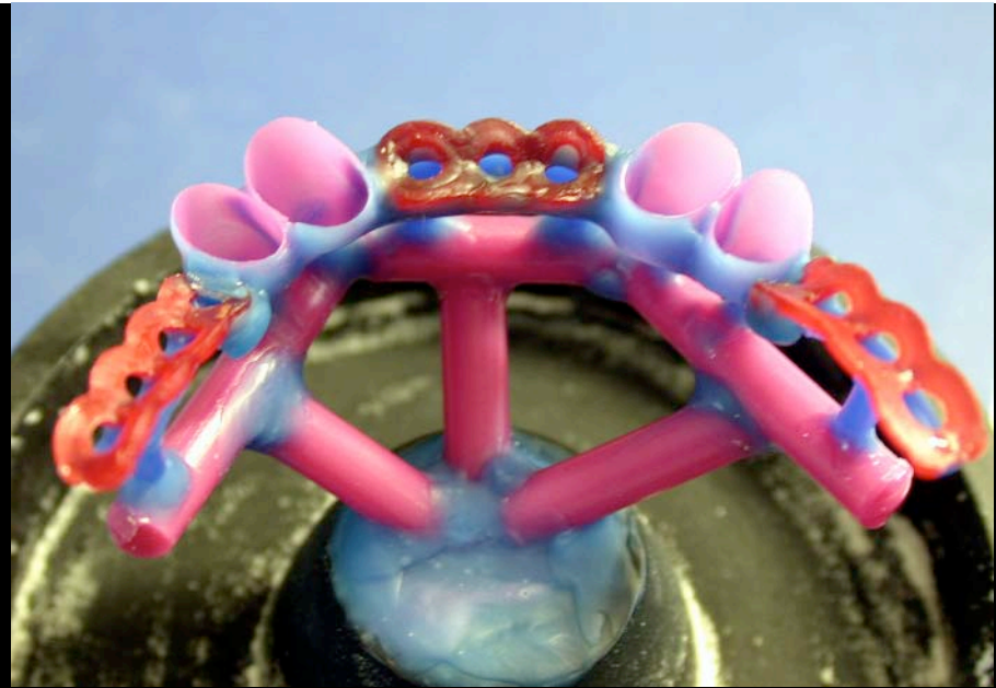
Wachmodellation in der Muffel
