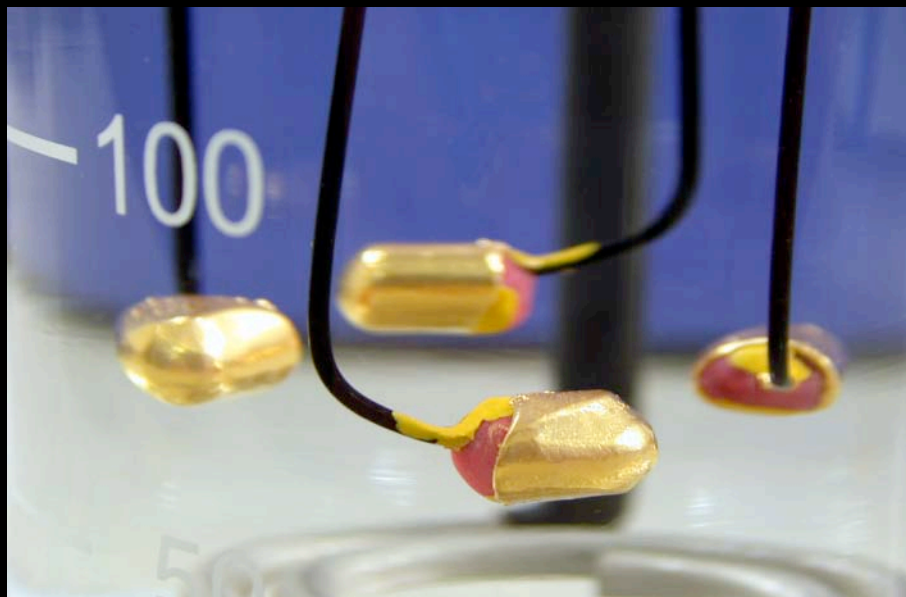
Galvanisierte Sekundärteile im Galvanokopf...
