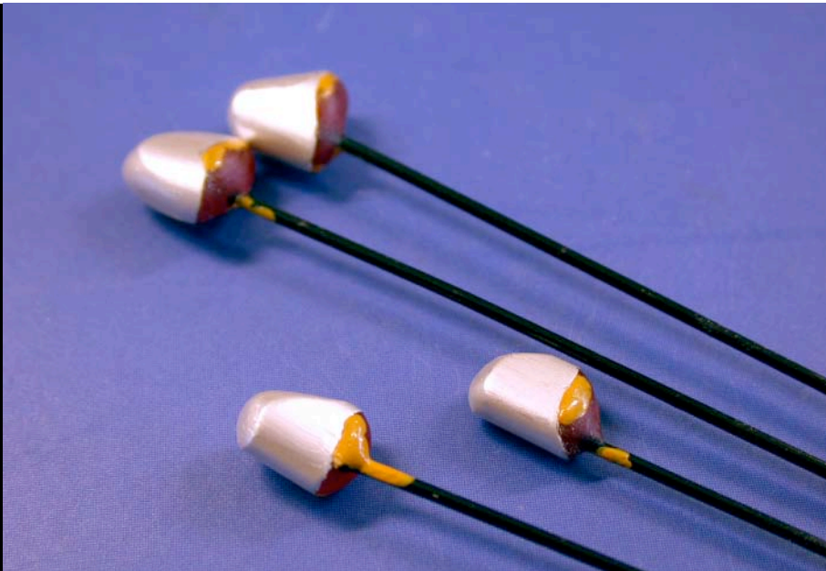
Primärteile mit Silberleitlack bestrichen, gefüllt mit Resin und kontaktiert
